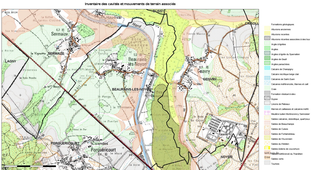
Illustration 2 : carte synthétique des formations argileuses et marneuses sur la commune de Beurains Les Noyon
