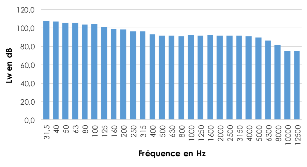
Figure 8. Graphe des niveaux de puissance acoustique d'une Nordex N117 – 3,6 MW (STE) par bande de tiers d'octave à la vitesse de 8 m/s (à la hauteur standardisée de 10 m)
