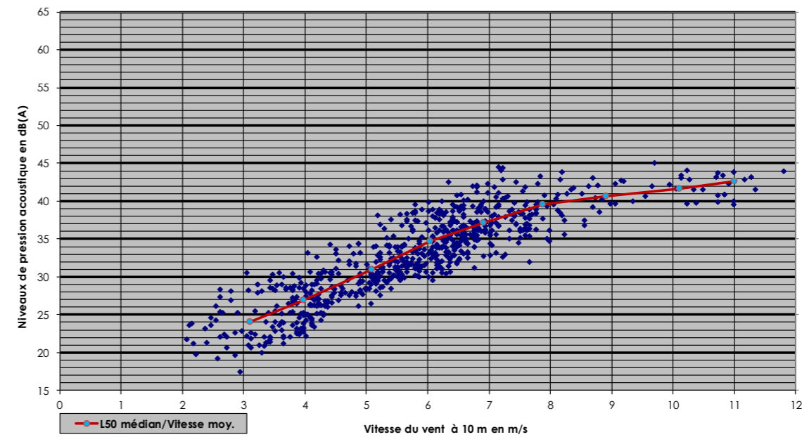
Niveaux de bruit résiduel mesurés de nuit en fonction du vent Puits-la-Vallée
