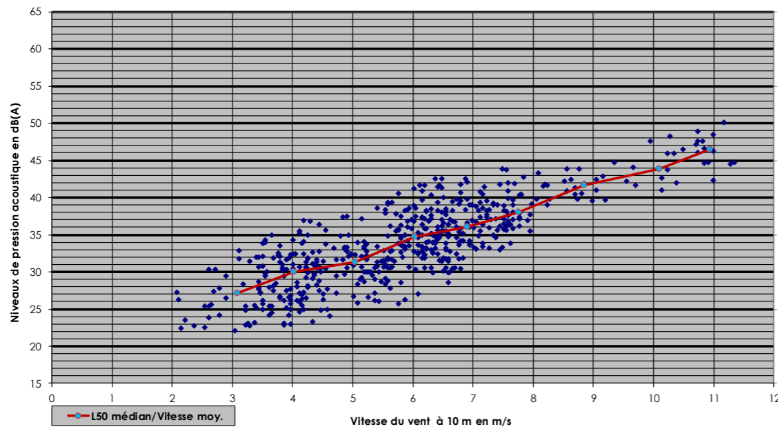
Niveaux de bruit résiduel mesurés de nuit en fonction du vent Petit Froissy
