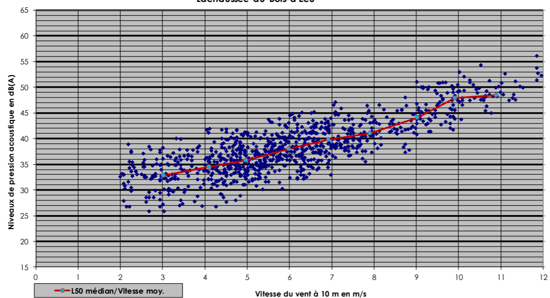
Niveaux de bruit résiduel mesurés de jour en fonction du vent Lachaussée-du-Bois-d'Écu
