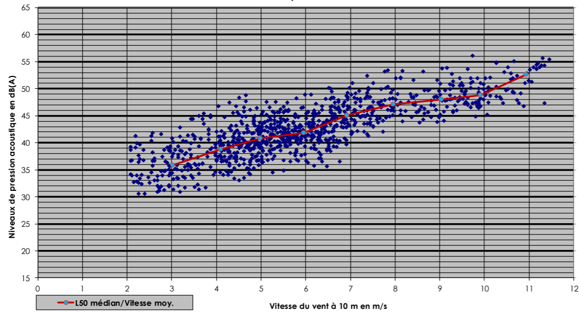
Niveaux de bruit résiduel mesurés de jour en fonction du vent Petit Froissy
