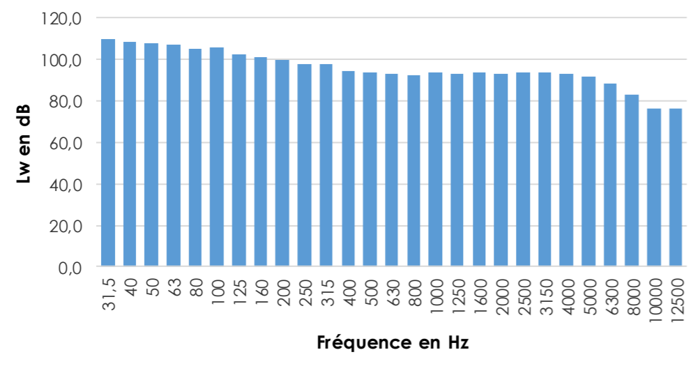
Figure 7. Graphe des niveaux de puissance acoustique d'une Nordex N117 – 3,6 MW (SANS SERRATIONS) par bande de tiers d'octave à la vitesse de 8 m/s (à la hauteur standardisée de 10 m)
