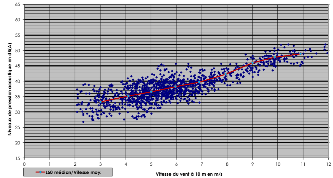
Niveaux de bruit résiduel mesurés de jour en fonction du vent Puits-la-Vallée
