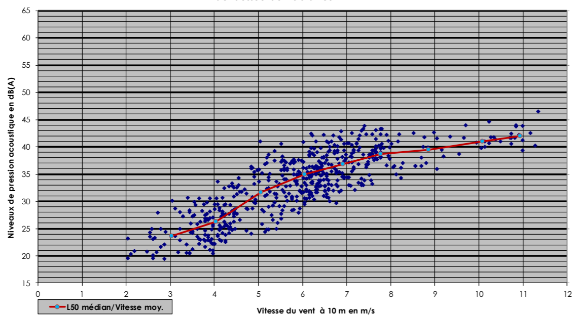
Niveaux de bruit résiduel mesurés de nuit en fonction du vent Lachaussée-du-Bois-d'Écu
