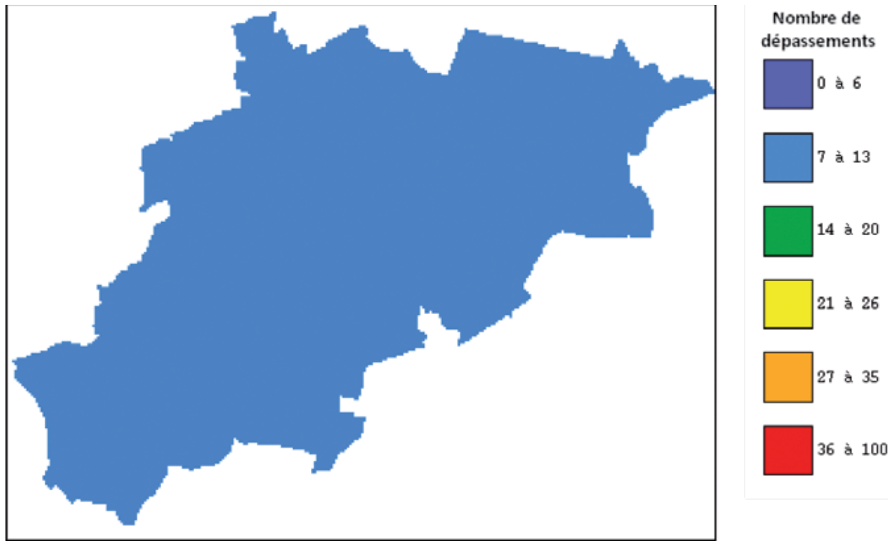
illustration 34 : Tendancier 2020 - Nombre de jours de dépassements de la valeur limite journalière en PM10 (source ATMO Picardie)
