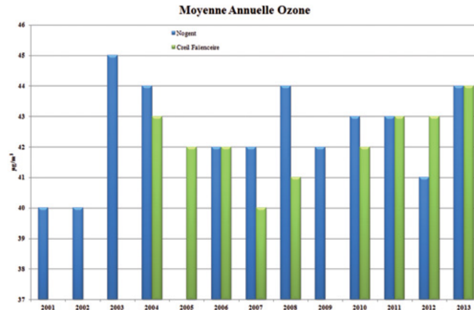
Illustration 35 : Evolution des concentrations annuelles en O 3 - Département de l'Oise - [Source Atmo Picardie]
