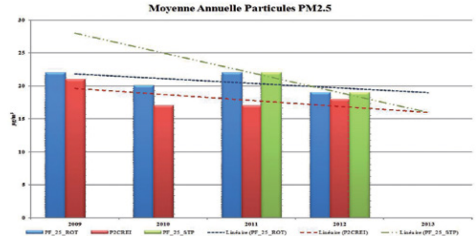
Illustration 38 : Evolution des concentrations annuelles en PM2,5 - Département de l'Oise - (Source Atmo Picardie)
