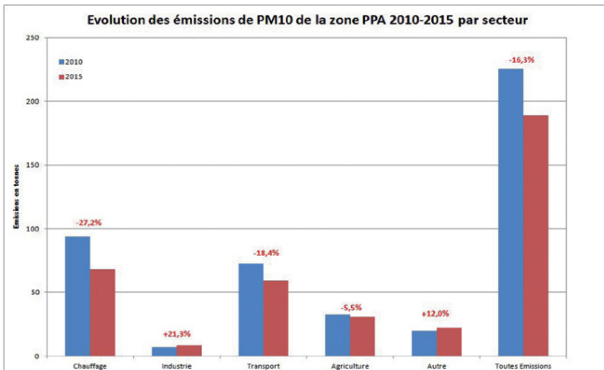
Graphique 2010 - 2015. Scénarisation de la zone PPA 2015 - évolution des émissions de PM10 - Source ATMO Picardie
