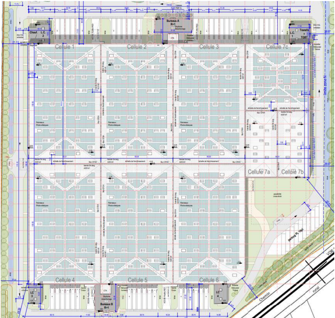
Figure 1 : Plan de masse du site
