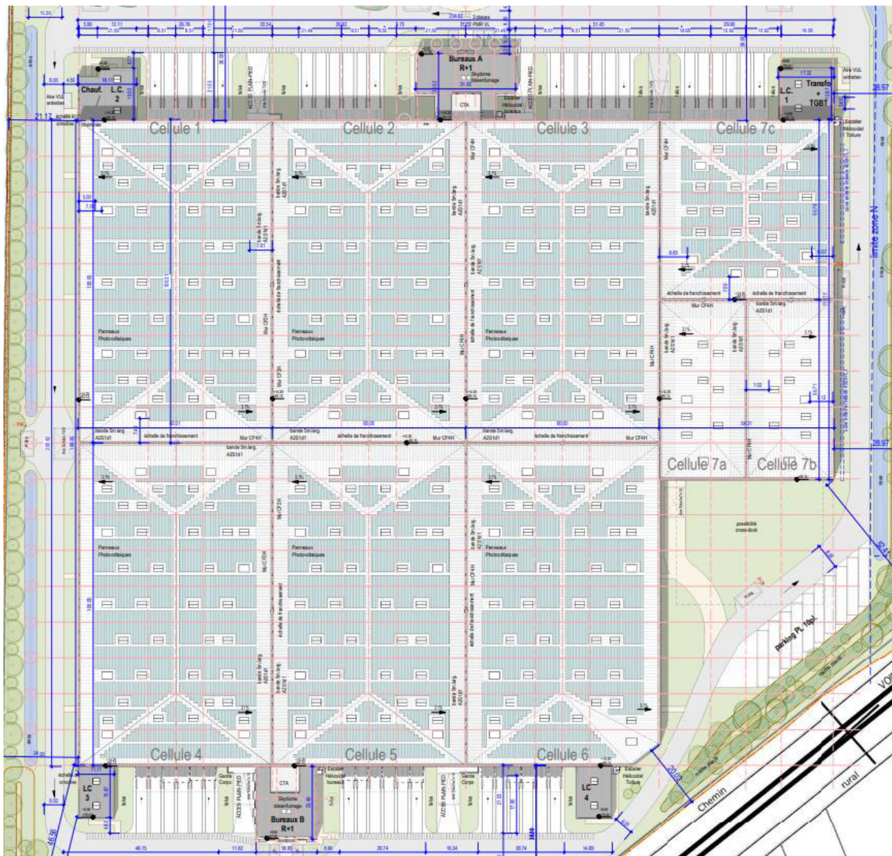
Figure 1: Plan de masse du site
