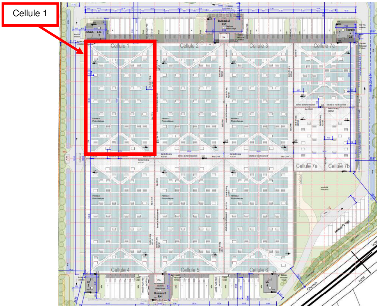
Figure 4: Découpage en cellule du site
